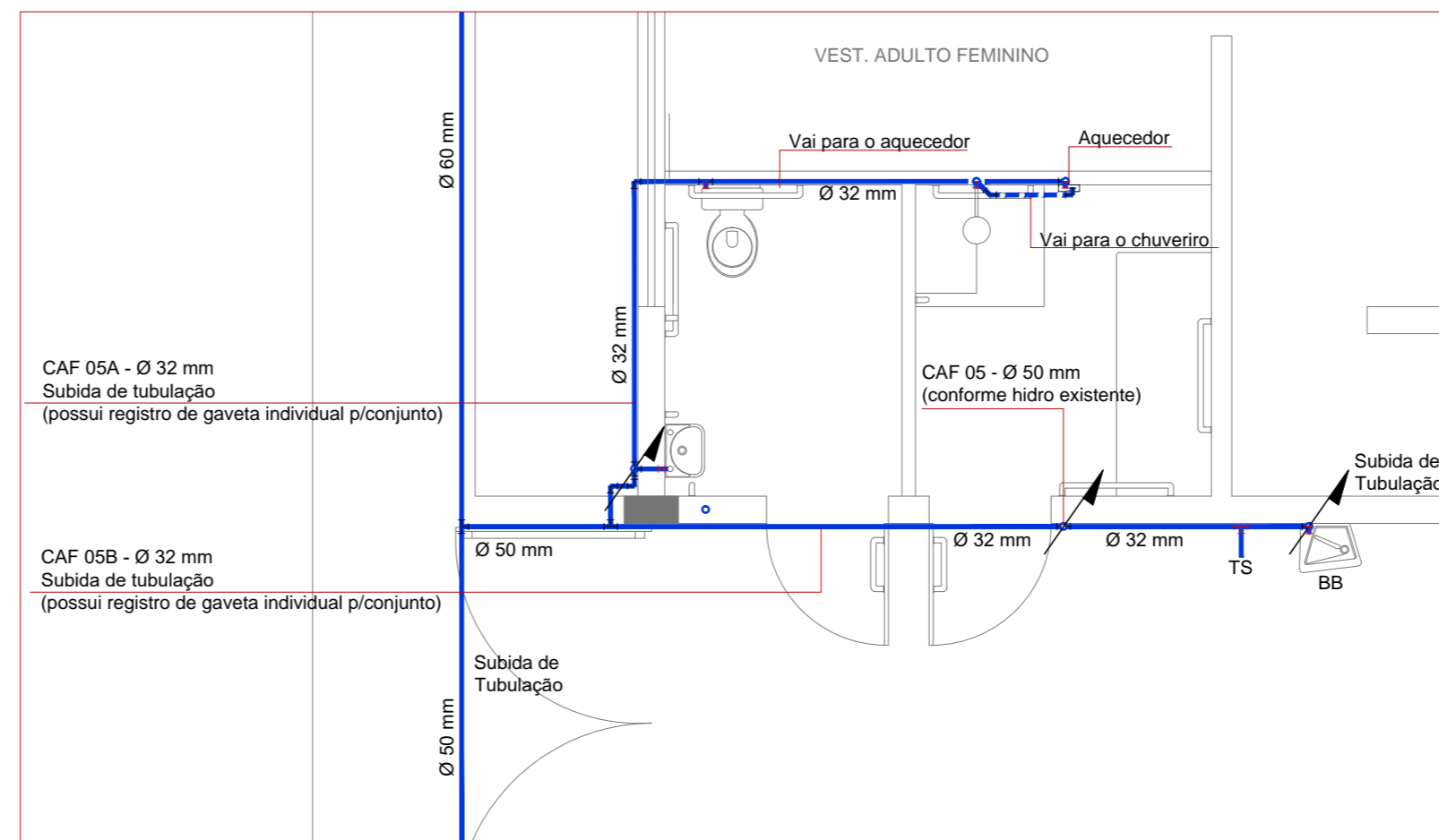
Planta Baixa Hidrossanitário Água Potável - Detalhe n° 02 ESCALA: 1/50
