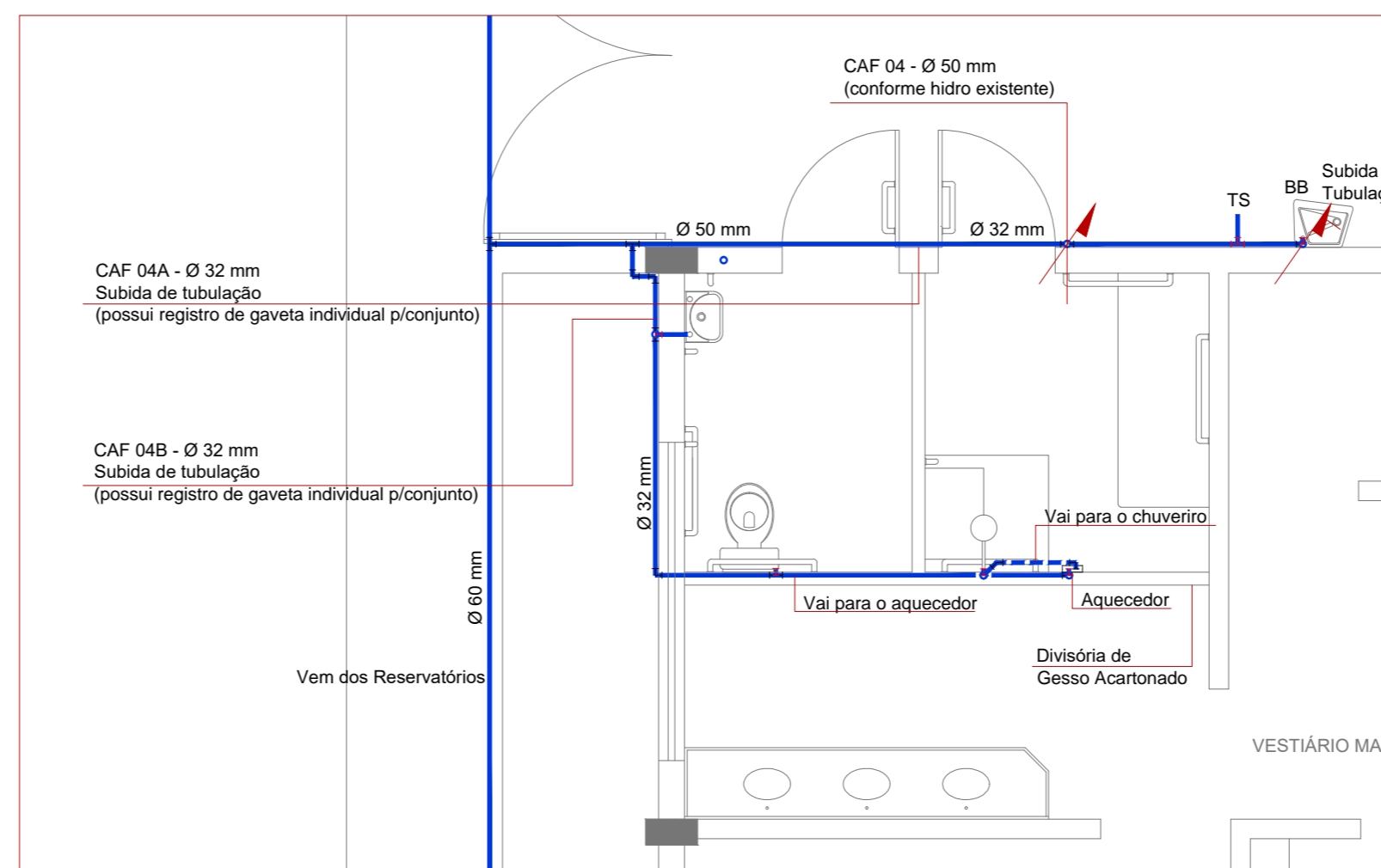
Planta Baixa Hidrossanitário Água Potável - Detalhe n° 03 ESCALA: 1/50
