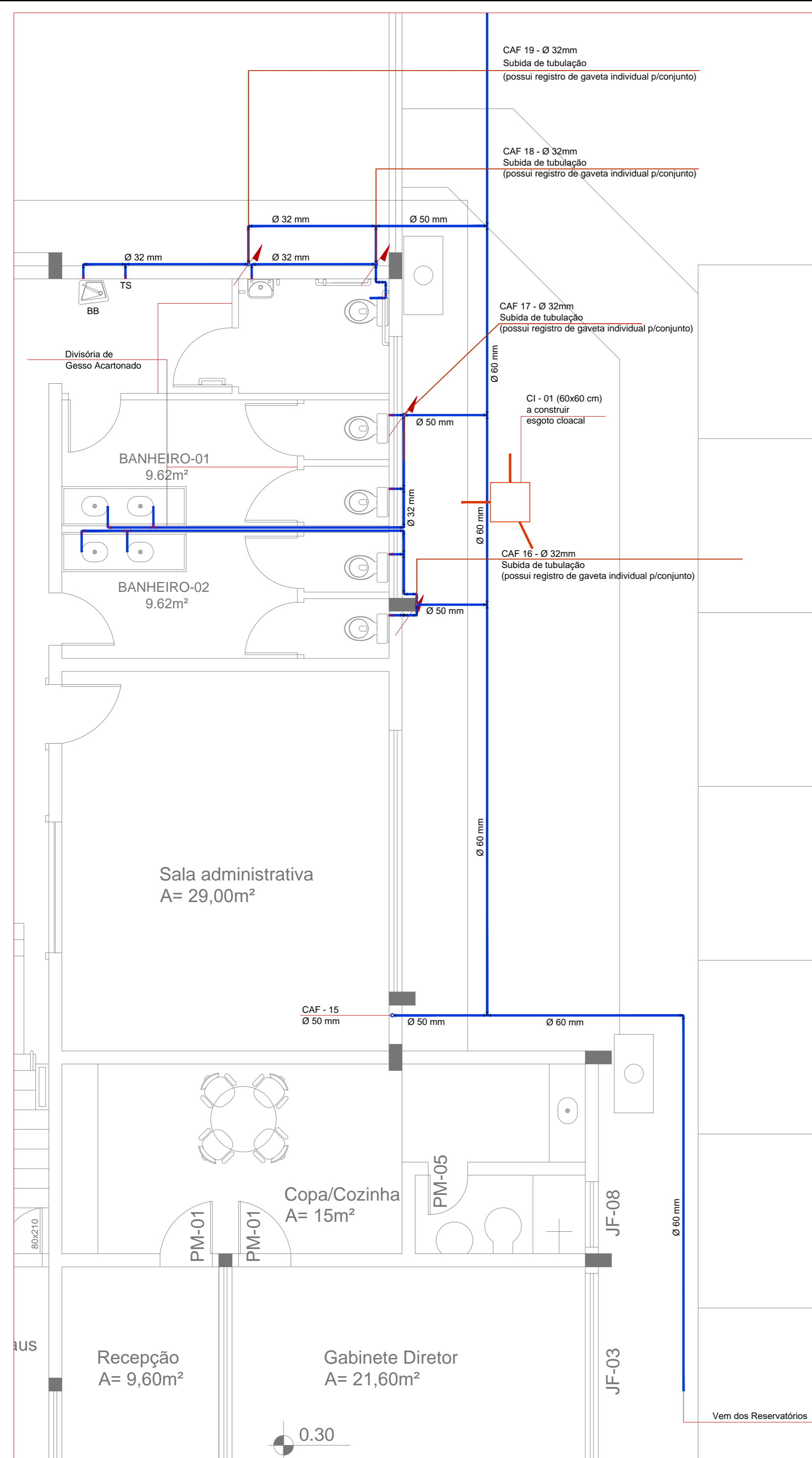
Planta Baixa Hidrossanitário Água Potável - Detalhe n° 01A ESCALA: 1/50
