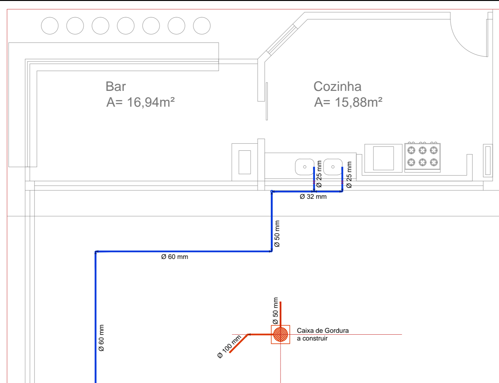
Planta Baixa Hidrossanitário Água Potável - Detalhe n° 01B ESCALA: 1/50
