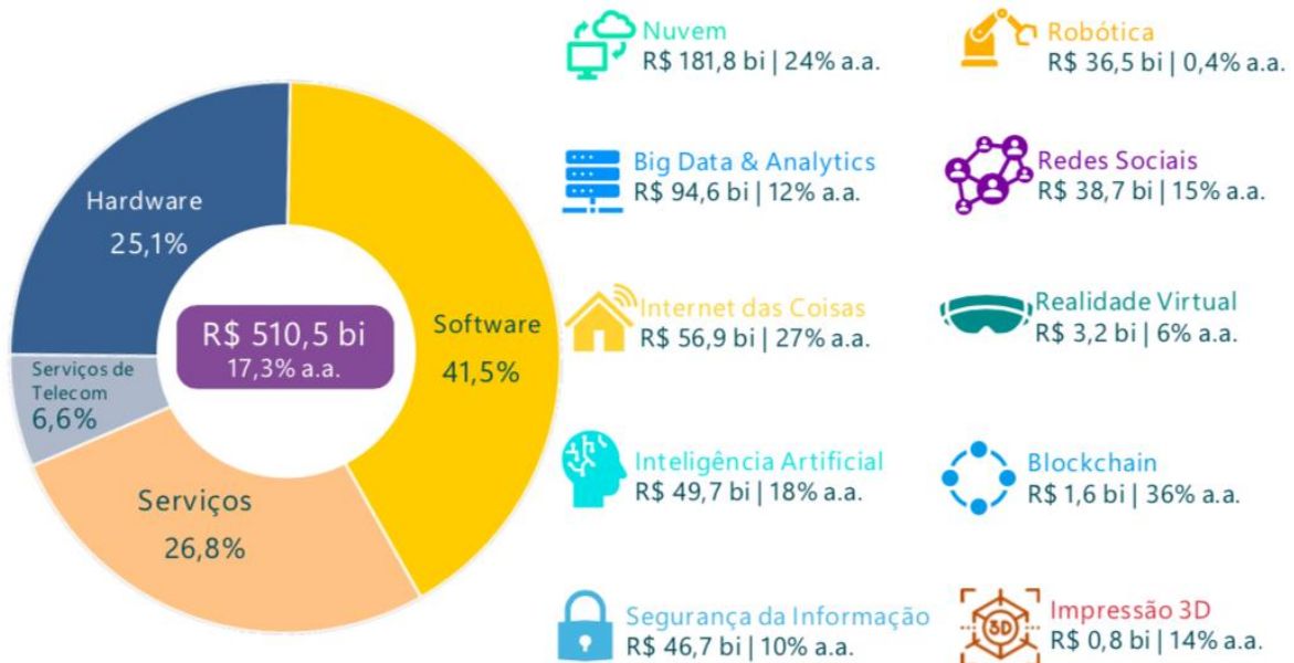
Figura 8 – Maiores montantes de investimentos em T.I. nos próximos anos
