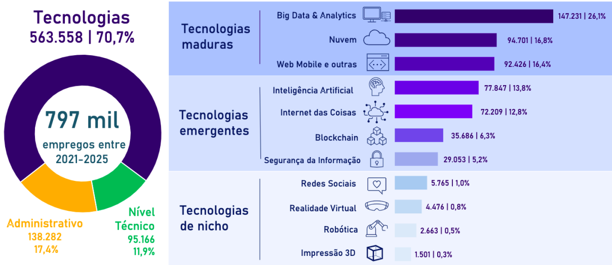
Figura 7 – Principais tecnologias geradoras de empregos nos próximos 5 anos
