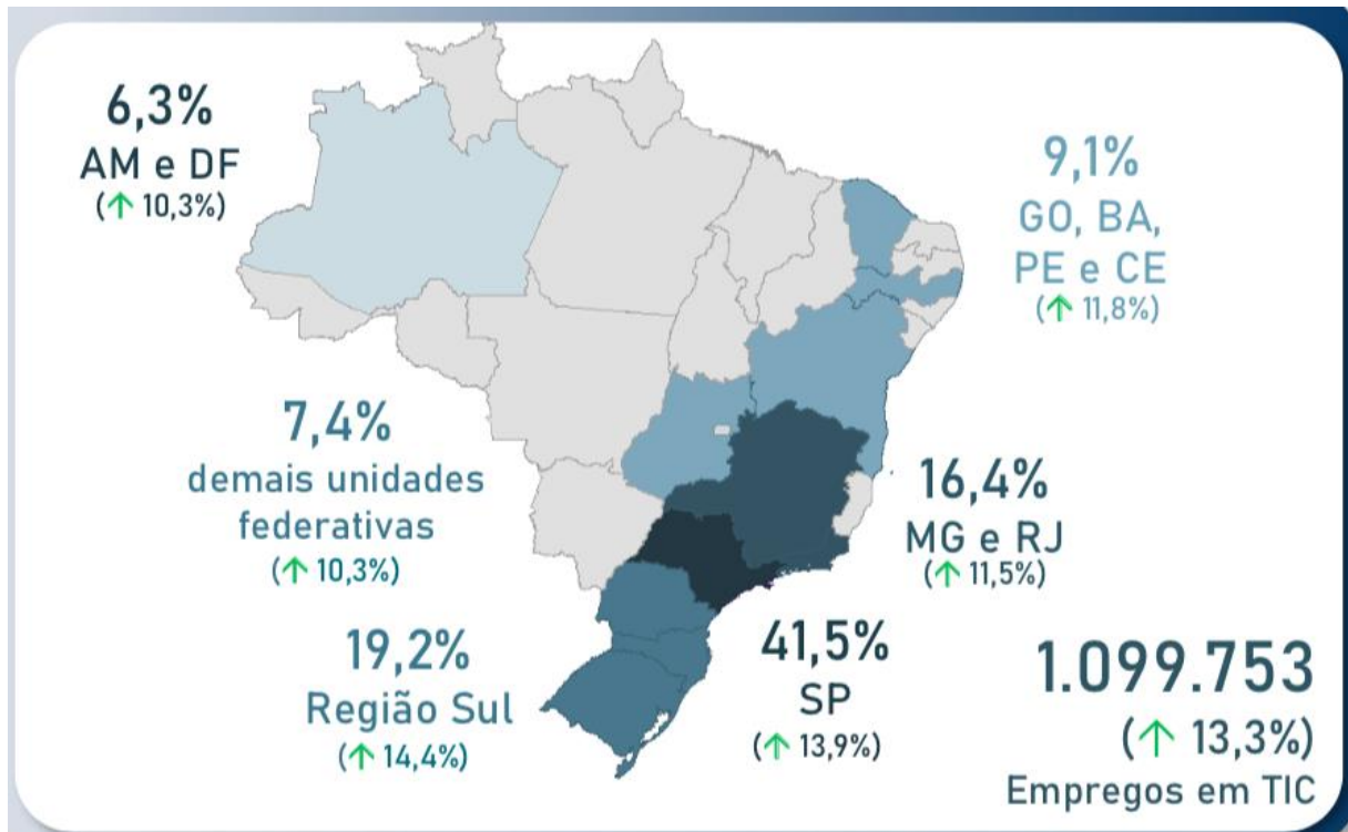
Figura 6 – Concentração de empregos na área de Tecnologia da Informação
